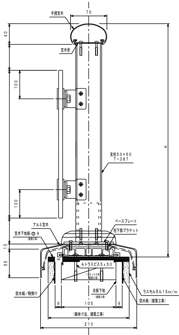
側面
