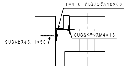
B部詳細
