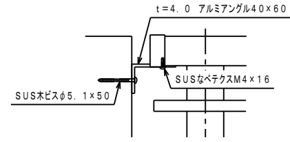
B部詳細
